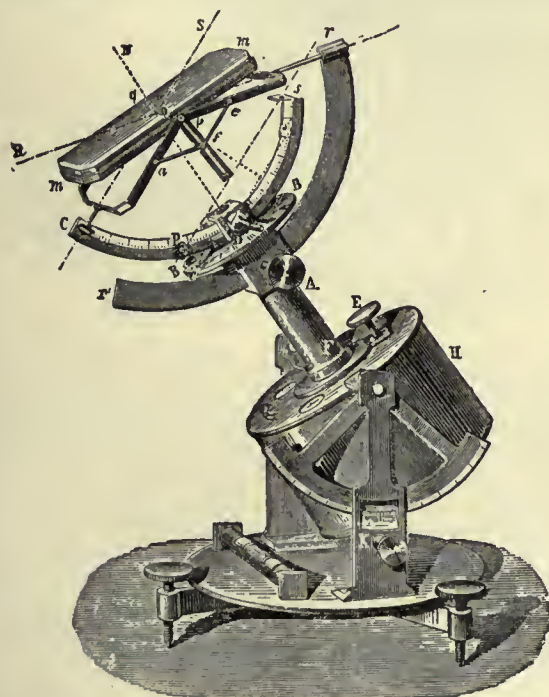
From Jamin and Bouty, Cours de physique , Gauthier-Villars. FIG. 3.—Silbermann's Heliostat.
